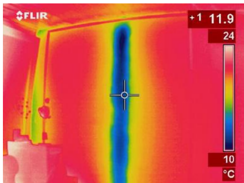
Toplotno neizolirani odtok meteorne vode z ravne strehe v notranji steni stavbe.
