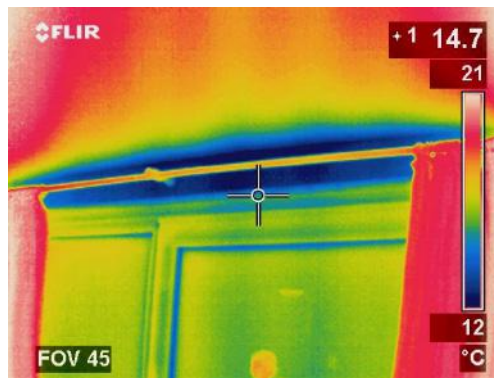
Izrazit toplotni most v območju preklade nad stavbnim pohištvom (posnetek z notranje strani).
