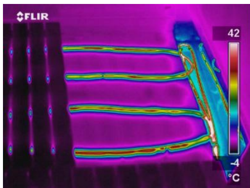
Termografski posnetek prosto položenih vodnikov električnega ogrevanja za taljenje snega pred izdelavo zaključnega pohodnega sloja.
