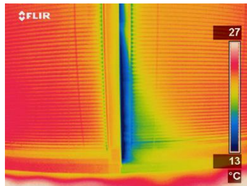
Termografski prikaz netesne pripire drsniških balkonskih vrat (posnetek z notranje strani).
