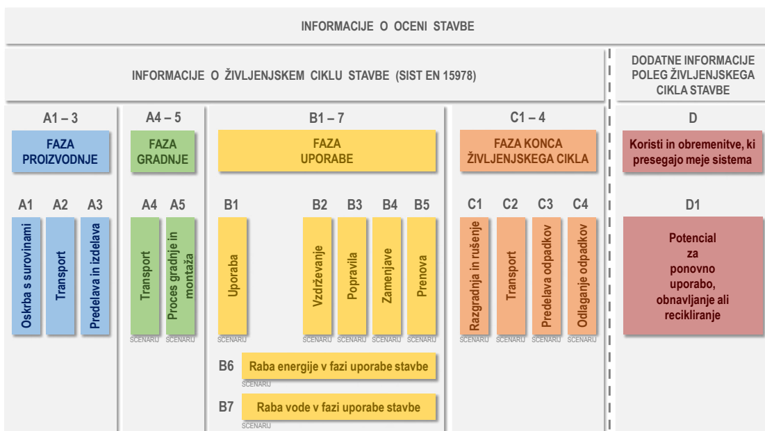
Slika 2. Faze življenjskega cikla stavbe, ki jih obravnavamo pri načrtovanju stavbe z mislijo na celotni življenjski cikel; Vir: LIFE IP CARE4CLIMATE
